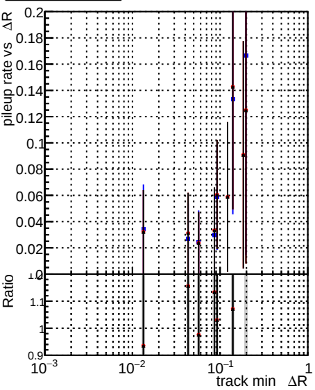
Legend: DQM original originalvector 1000evt, DQM fit cpeOK SORTR22 TESTOUTLIER5 1000evt, DQM fit cpeOK SORTR22 TESTOUTLIER6 1000evt
