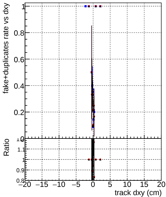
DQM_original_originalvector_1000evt DQM_fit_cpeOK_SORTRZ2_TESTOUTLIER5_1000evt DQM_fit_cpeOK_SORTRZ2_TESTOUTLIER6_1000evt
