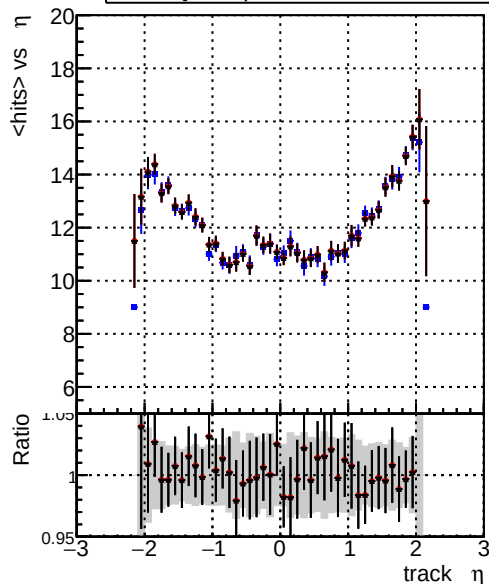
mean hits vs \eta — DQM_original_originalvector_1000evt — DQM_fit_cpeOK_SORTR22_TESTOUTLIER5_1000evt — DQM_fit_cpeOK_SORTR22_TESTOUTLIER6_1000evt
