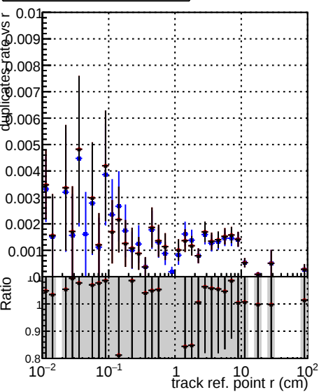
—■— DQM original originalvector 1000evt —●— DQM fit cpeOK SORTR22 TESTOUTLIER5 1000evt —+— DQM fit cpeOK SORTR22 TESTOUTLIER6 1000evt
