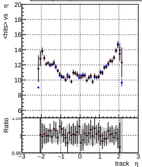
mean hits vs \eta — DQM_original_originalvector_1000evt — DQM_fit_cpeOK_SORTRZ2_TESTOUTLIER5_1000evt — DQM_fit_cpeOK_SORTRZ2_TESTOUTLIER6_1000evt
