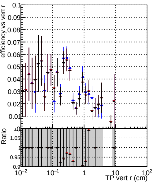
Efficiency vs TP vert r (cm) Legend: DQM_original_originalvector_1000evt DQM_fit_cpeOK_SORTRZ2_TESTOUTLIER5_1000evt DQM_fit_cpeOK_SORTRZ2_TESTOUTLIER6_1000evt
