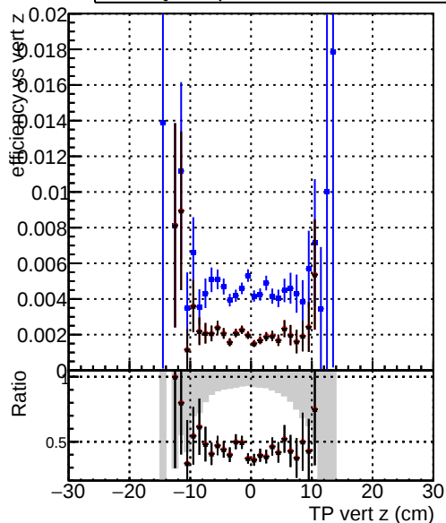
Efficiency vs. TP vert z (cm) Legend: - DQM_original_originalvector_1000evt (blue stars) - DQM_fit_cpeOK_SORTRZ2_TESTOUTLIER5_1000evt (red line) - DQM_fit_cpeOK_SORTRZ2_TESTOUTLIER6_1000evt (black line)
