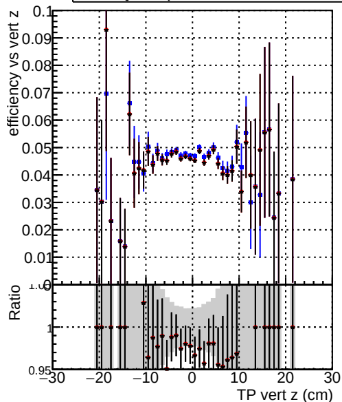
Efficiency —●— DQM_original_originalvector_1000evt —●— DQM_fit_cpeOK_SORTRZ2_TESTOUTLIER5_1000evt —●— DQM_fit_cpeOK_SORTRZ2_TESTOUTLIER6_1000evt
