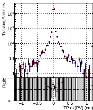
N of simulated tracks vs dz(PV) 0 100 1 100 2 100 3 100 4 100 5 100 6 100 7 100 8 100 9 100 10 100 11 100 12 100 13 100 14 100 15 100 16 100 17 100 18 100 19 100 20 100 21 100 22 100 23 100 24 100 25 100 26 100 27 100 28 100 29 100 30 100 31 100 32 100 33 100 34 100 35 100 36 100 37 100 38 100 39 100 40 100 41 100 42 100 43 100 44 100 45 100 46 100 47 100 48 100 49 100 50 100 51 100 52 100 53 100 54 100 55 100 56 100 57 100 58 100 59 100 60 100 61 100 62 100 63 100 64 100 65 100 66 100 67 100 68 100 69 100 70 100 71 100 72 100 73 100 74 100 75 100 76 100 77 100 78 100 79 100 80 100 81 100 82 100 83 100 84 100 85 100 86 100 87 100 88 100 89 100 90 100 91 100 92 100 93 100 94 100 95 100 96 100 97 100 98 100 99 100 100 100
