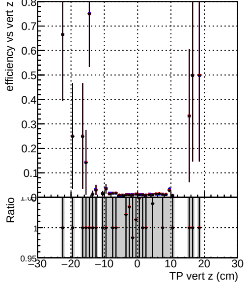
Efficiency vs vert z —●— DQM_original_originalvector_1000evt —●— DQM_fit_cpeOK_SORTRZ2_TESTOUTLIER5_1000evt —●— DQM_fit_cpeOK_SORTRZ2_TESTOUTLIER6_1000evt
