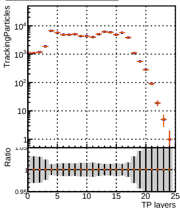
N of sim DQM_fit_cpeOK_SORTRZ2_TESTOUTLIER6_1000evt DQM_fit_cpeOK_SORTRZ2_TESTOUTLIER6_getS_1000evt
