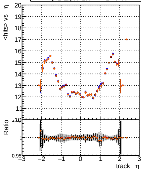
mean hits vs \eta — DQM_fit_cpeOK_SORTRZ2_TESTOUTLIER5_1000evt — DQM_fit_cpeOK_SORTRZ2_TESTOUTLIER6_1000evt — DQM_fit_cpeOK_SORTRZ2_TESTOUTLIER6_getS_1000evt
