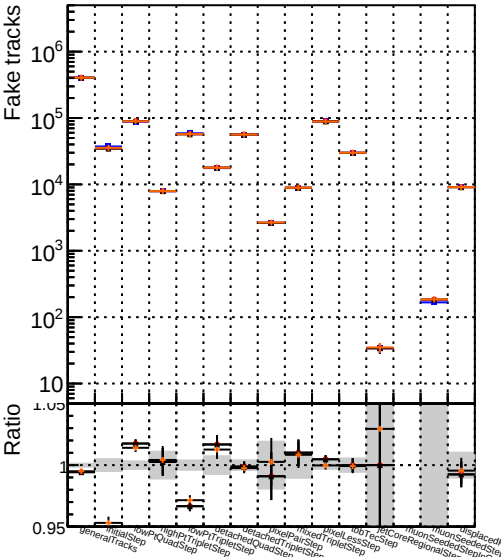
■ DQM original originalvector 1000evt ■ DQM fit cpeOK_SORTRZ2_TESTOUTLIER5_1000evt ■ DQM fit cpeOK_SORTRZ2_TESTOUTLIER6_1000evt ■ DQM fit cpeOK_SORTRZ2_TESTOUTLIER6_getS_1000evt
