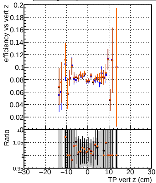
Efficiency vs vert z DOM original originalvector 1000evt DOM_fit_cpeOK_SORTRZ2_TESTOUTLIER5_1000evt DOM_fit_cpeOK_SORTRZ2_TESTOUTLIER6_1000evt DOM_fit_cpeOK_SORTRZ2_TESTOUTLIER6_getS_1000evt
