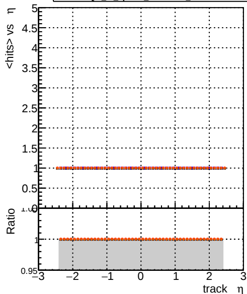
mean hits — DQM original originalvector 1000evt — DQM_fit_cpeOK_SORTRZ2_TESTOUTLIER5_1000evt — DQM_fit_cpeOK_SORTRZ2_TESTOUTLIER6_1000evt — DQM_fit_cpeOK_SORTRZ2_TESTOUTLIER6_getS_1000evt
