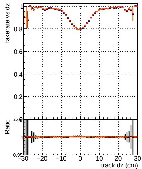
Fake rate vs d DOM original originalvector 1000evt DOM fit cpeak SORTR22 TESTOUTLIER5 1000evt DOM fit cpeak SORTR22 TESTOUTLIER6 1000evt
