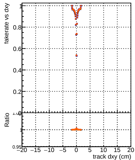
Fake rate vs d DOM original originalvector 1000evt DOM fit cpeak SORTR22 TESTOUTLIER5 1000evt DOM fit cpeak SORTR22 TESTOUTLIER6 1000evt
