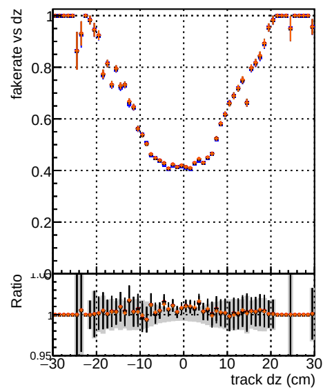
Fake rate vs dz BGM original-originalvector 1000evt BGM IL CBOOK SORTRZZ TESTOUTLIER 1000evt BGM IL CBOOK SORTRZZ TESTOUTLIER 995 1000evt
