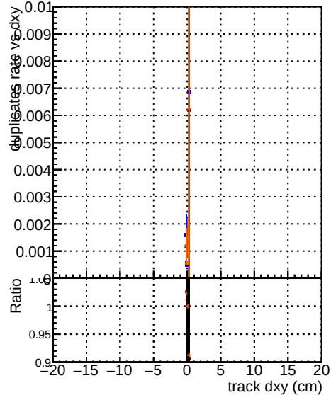
STOUTLIER6=1000evt
