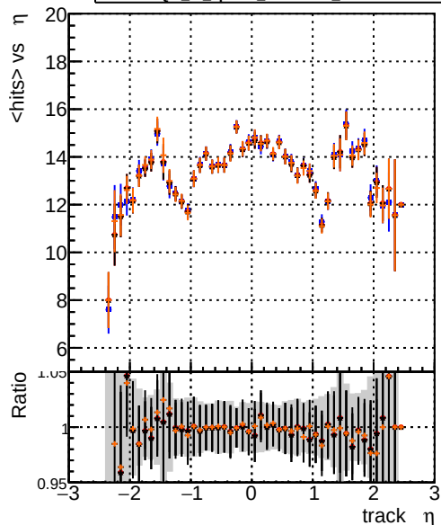
mean hit \eta DOM original originalvector 1000evt DOM_fit_cpeOK_SORTRZ2_TESTOUTLIER5_1000evt DOM_fit_cpeOK_SORTRZ2_TESTOUTLIER6_1000evt DOM_fit_cpeOK_SORTRZ2_TESTOUTLIER6_getS_1000evt
