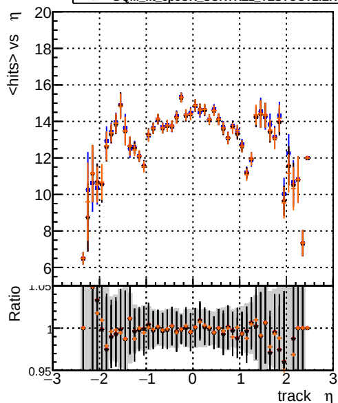
mean hits vs \eta DOM originalvector 1000evt DOM_fit_cpeOK_SORTR22_TESTOUTLIER5_1000evt DOM_fit_cpeOK_SORTR22_TESTOUTLIER6_1000evt DOM_fit_cpeOK_SORTR22_TESTOUTLIER6_getS_1000evt
