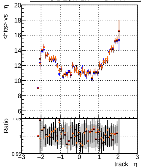
mean hits vs \eta DOM original originalvector 1000evt DOM_fit_cpeOK_SORTRZ2_TESTOUTLIER5_1000evt DOM_fit_cpeOK_SORTRZ2_TESTOUTLIER6_1000evt DOM_fit_cpeOK_SORTRZ2_TESTOUTLIER6_getS_1000evt
