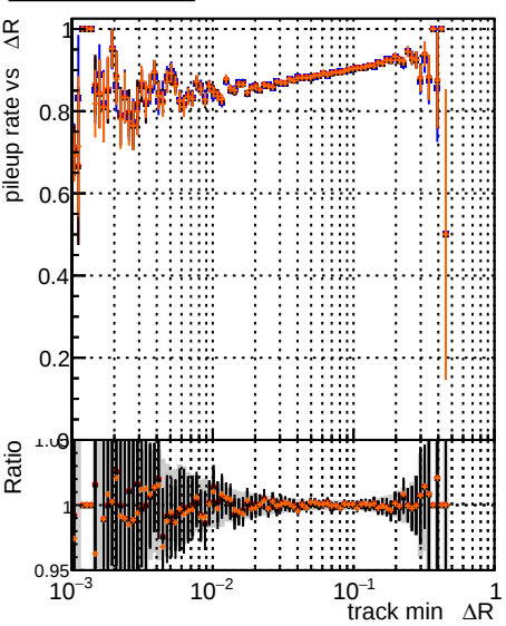
Legend: - DOM original original vector 1000evt - DOM fit cpeok SORTBZZ TESTOUTLIER5 1000evt - DOM fit cpeok SORTBZZ TESTOUTLIER6 1000evt - DOM fit cpeok SORTBZZ TESTOUTLIER8 gets 1000evt
