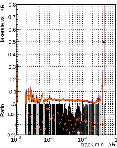
Legend: - DOM original original vector 1000evt - DOM fit cpeok SORTBZZ TESTOUTLIER5 1000evt - DOM fit cpeok SORTBZZ TESTOUTLIER6 1000evt - DOM fit cpeok SORTBZZ TESTOUTLIER8 gets 1000evt
