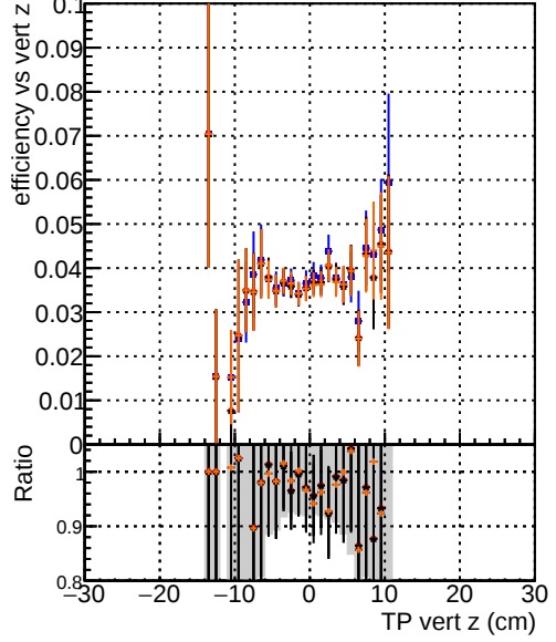
Efficiency vs vert z — DQM original originalvector 1000evt — DQM fit cpeOK_SORTRZ2_TESTOUTLIER5 1000evt — DQM fit cpeOK_SORTRZ2_TESTOUTLIER6 1000evt — DQM fit cpeOK_SORTRZ2_TESTOUTLIER6 gets 1000evt
