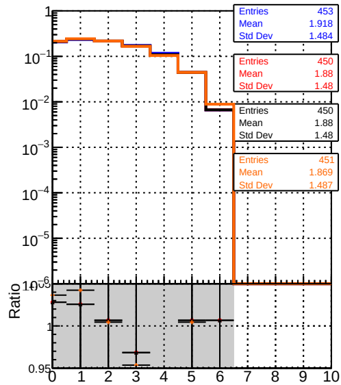
DOM original originalvector 1000evt DOM_fit_cpeOK_SORTRZ2_TESTOUTLIER5_1000evt DOM_fit_cpeOK_SORTRZ2_TESTOUTLIER6_1000evt DOM_fit_cpeOK_SORTRZ2_TESTOUTLIER6_getS_1000evt
