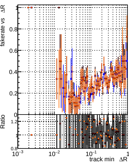
Fake rate vs \Delta R(\text{track, jet}) DQM original original vector 1000evt DQM fit cpeok SORTBZZ TESTOUTLIER5 1000evt DQM fit cpeok SORTBZZ TESTOUTLIER6 gets 1000evt
