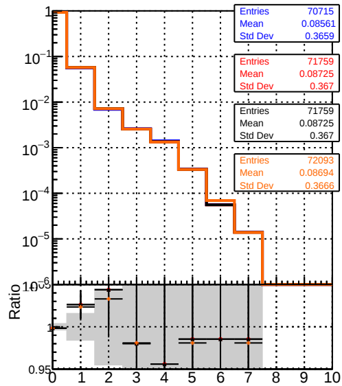
DOM_fit_cpeOK_SORTRZ2_TESTOUTLIER5_1000evt DOM_fit_cpeOK_SORTRZ2_TESTOUTLIER6_1000evt DOM_fit_cpeOK_SORTRZ2_TESTOUTLIER6_getS_1000evt mean hits
