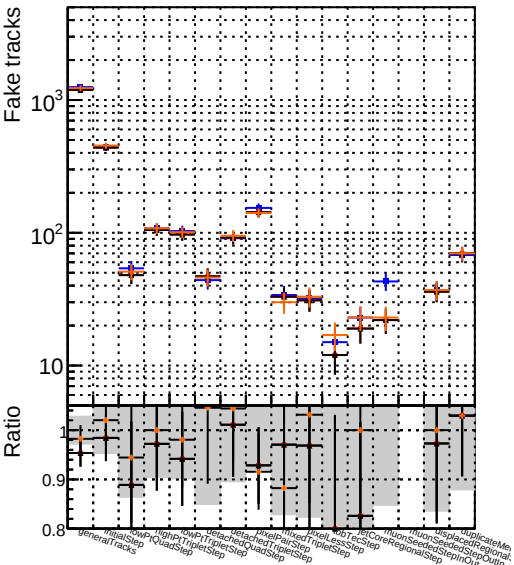
Numbe —▲— DQM_fit_cpeOK_SORTRZ2_TESTOUTLIER6_1000evt —◆— DQM_fit_cpeOK_SORTRZ2_TESTOUTLIER6_getS_1000evt
