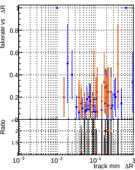
Fake rate vs ΔR(track, jet) DQM original 1000evt DQM fit 1000evt DQM fit cpeok 1000evt DQM fit cpeok sorted 1000evt DQM original 1000evt DQM fit 1000evt DQM fit cpeok 1000evt DQM fit cpeok sorted 1000evt DQM original 1000evt DQM fit 1000evt DQM fit cpeok 1000evt DQM fit cpeok sorted 1000evt
