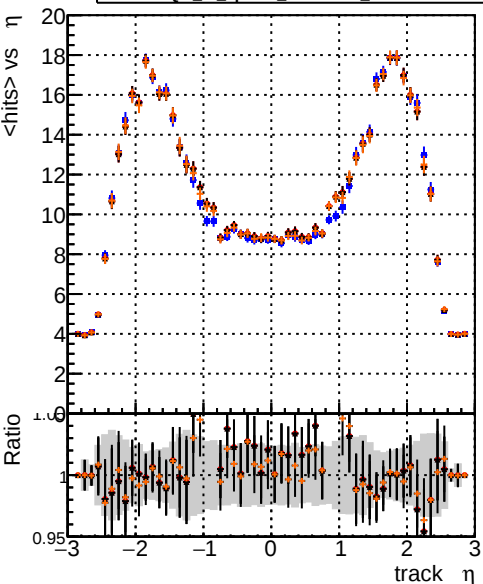
mean hit DOM_original originalvector 1000evt DOM_fit_cpeOK_SORTRZ2_TESTOUTLIER5_1000evt DOM_fit_cpeOK_SORTRZ2_TESTOUTLIER6_1000evt DOM_fit_cpeOK_SORTRZ2_TESTOUTLIER6_getS_1000evt
