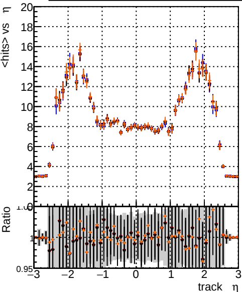
mean hit \eta DOM_original originalvector 1000evt DOM_fit_cpeOK_SORTRZ2_TESTOUTLIER5_1000evt DOM_fit_cpeOK_SORTRZ2_TESTOUTLIER6_1000evt DOM_fit_cpeOK_SORTRZ2_TESTOUTLIER6_getS_1000evt
