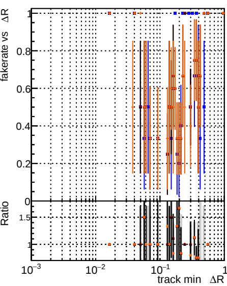
Fake rate vs \Delta R(\text{track, jet}) DQM original original vector 1000evt DOM fit cpeok SORTBZZ TESTOUTLIER5 1000evt DOM fit cpeok SORTBZZ TESTOUTLIER6 gets 1000evt
