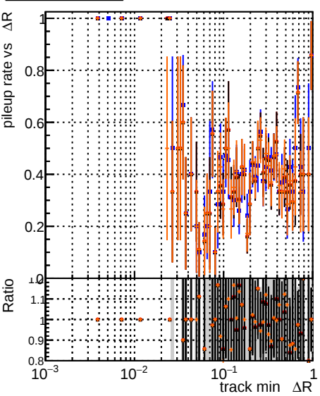
DOM original original vector 1000evt DOM fit cpeok sort RZ2 TESTOUTLIER5 1000evt DOM fit cpeok sort RZ2 TESTOUTLIER6 gets 1000evt
