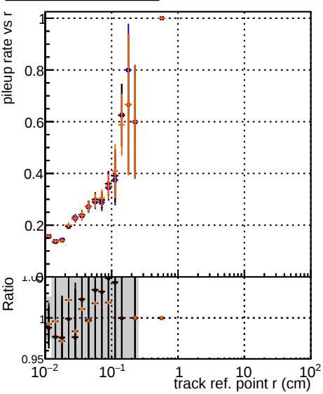
—•— BQM original original vector 1000evt —•— BQM fit cpeak SORTRZ2 TESTOUTLIER5 1000evt —•— BQM fit cpeak SORTRZ2 TESTOUTLIER6 1000evt —•— BQM fit cpeak SORTRZ2 TESTOUTLIER8 gets 1000evt
