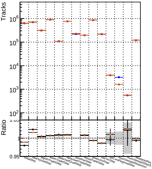
Number Legend DOM original originalvector 1000evt DOM fit cpeOK SORTRZ2 TESTOUTLIER5 1000evt DOM fit cpeOK SORTRZ2 TESTOUTLIER6 1000evt DOM fit cpeOK SORTRZ2 TESTOUTLIER6 getS 1000evt
