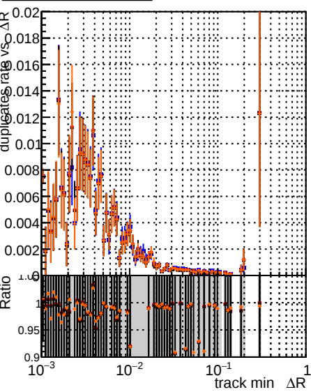
Legend: - \Delta R original original vector 1000evt - \Delta R fit cpeak SORTBZZ TESTOUTLIER5 1000evt - \Delta R fit cpeak SORTBZZ TESTOUTLIER6 gets 1000evt
