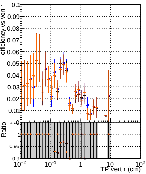
Efficiency vs TP vert r (cm) Legend: DOM original originalvector 1000evt DOM_fit_cpeOK_SORTRZ2_TESTOUTLIER5_1000evt DOM_fit_cpeOK_SORTRZ2_TESTOUTLIER6_1000evt DOM_fit_cpeOK_SORTRZ2_TESTOUTLIER6_getS_1000evt
