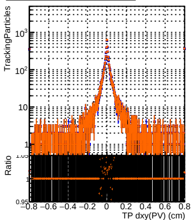
N of sim DQM_original_originalvector_1000evt DQM_fit_cpeOK_SORTRZ2_TESTOUTLIER5_1000evt DQM_fit_cpeOK_SORTRZ2_TESTOUTLIER6_1000evt DQM_fit_cpeOK_SORTRZ2_TESTOUTLIER6_getS_1000evt
