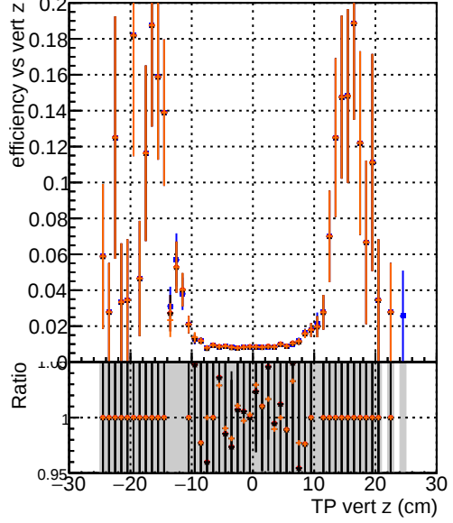
Efficiency vs vert z —●— DOM original originalvector 1000evt —●— DOM_fit_cpeOK_SORTRZ2_TESTOUTLIER5_1000evt —●— DOM_fit_cpeOK_SORTRZ2_TESTOUTLIER6_1000evt —●— DOM_fit_cpeOK_SORTRZ2_TESTOUTLIER6_getS_1000evt
