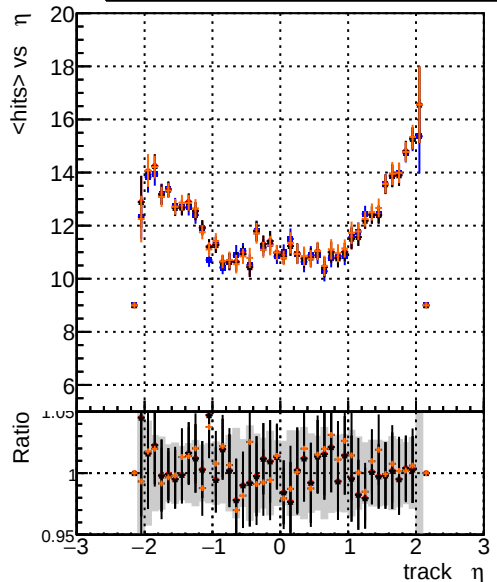
DOM original originalvector 1000evt DOM_fit_cpeOK_SORTRZ2_TESTOUTLIER5_1000evt DOM_fit_cpeOK_SORTRZ2_TESTOUTLIER6_1000evt DOM_fit_cpeOK_SORTRZ2_TESTOUTLIER6_getS_1000evt
