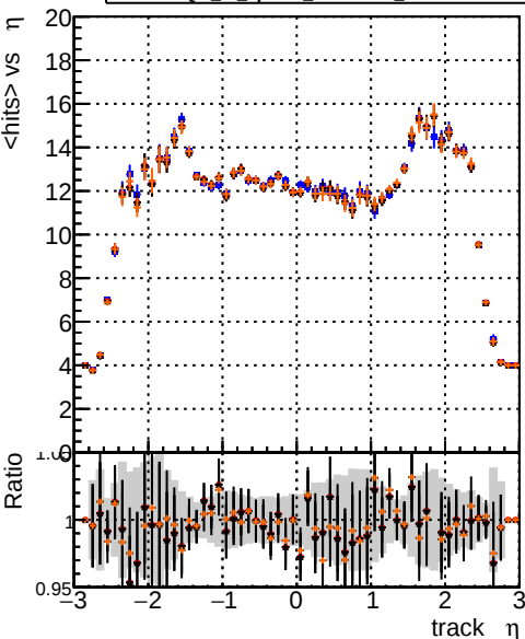
mean hits vs \eta DOM originalvector 1000evt DOM_fit_cpeOK_SORTRZ2_TESTOUTLIER5_1000evt DOM_fit_cpeOK_SORTRZ2_TESTOUTLIER6_1000evt DOM_fit_cpeOK_SORTRZ2_TESTOUTLIER6_getS_1000evt
