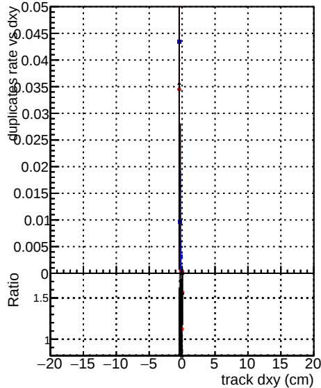
ttbar-phase1-newgeom
