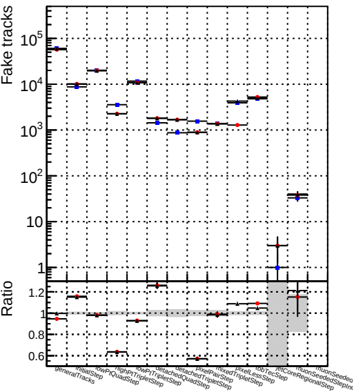
Number —■— DQMstep3_ZToEE_CKF —●— DQMstep3_ZToEE_default —★— DQMstep3_ZToEE_ckfPixelLess
