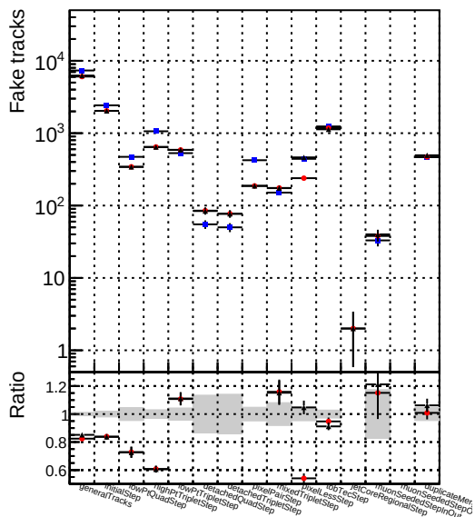
—●— DQMstep3_ZToEE_CKF —●— DQMstep3_ZToEE_default —●— DQMstep3_ZToEE_ckfPixelLess
