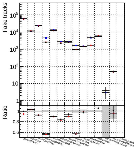
Number 1 ● DQMstep3_ZToEE_default 2 ▲ DQMstep3_ZToEE_ckfPixelLess
