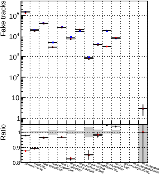
Number —■— DQMstep3_ZToEE_CKF —●— DQMstep3_ZToEE_default —★— DQMstep3_ZToEE_ckfPixelLess
