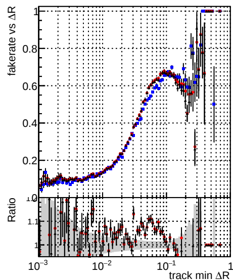
—●— DQMstep3_ZToEE_CKF —●— DQMstep3_ZToEE_default —●— DQMstep3_ZToEE_ckfPixelLess
