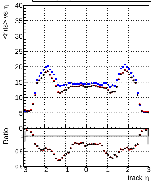
— DQMstep3_ZToEE_CKF — DQMstep3_ZToEE_default — DQMstep3_ZToEE_ckfPixelLess
