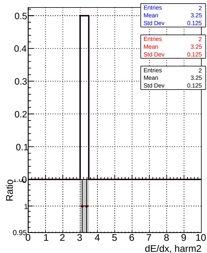
dE/dx estimator 1
