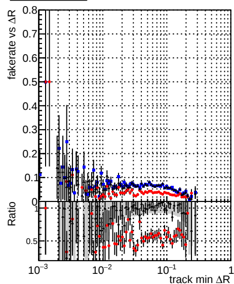
Legend: DQMstep3_ZToEE_CKF (blue circles) DQMstep3_ZToEE_default (red circles) DQMstep3_ZToEE_ckfPixelLess (black circles)
