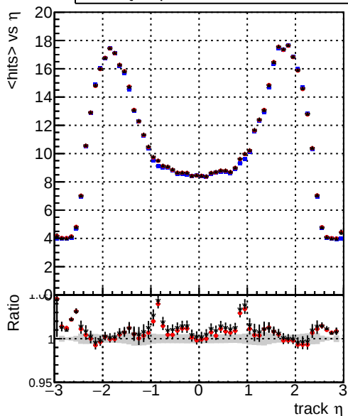
DQMstep3_ZToEE_CKF DQMstep3_ZToEE_default DQMstep3_ZToEE_ckfPixelLess mean hit
